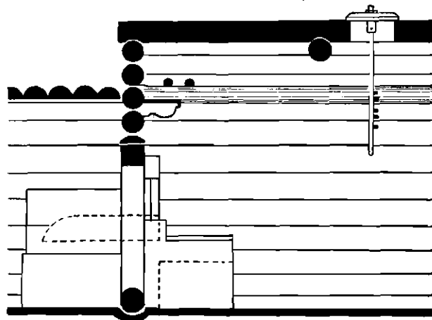
Ryc. 20. Konstrukcja urządzenia wentylacyjnego w kurnej chałupie, Zubrzyca Górna.
