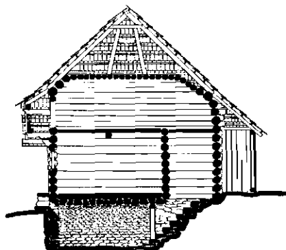
Ryc. 10. Przekrój poprzeczny przez chałupę Czopa z Zubrzycy Górnej.
