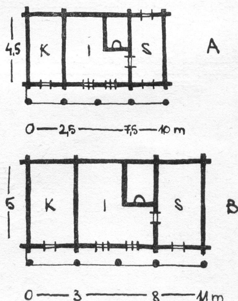
Il. 3. Plany bojkowski chałup centralnych: A — 1792 r., Orawczyk; B — pocz. XIX w., Lichobory.
