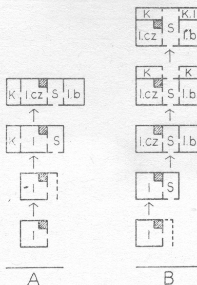
Il. 11. Chałupa o układzie: stajnia-sień-izba-komora, poł. XIX w., Nienadowa Dolna k. Dubiecka. Il. 12. Dwie linie rozwojowe domu na Podhalu.
